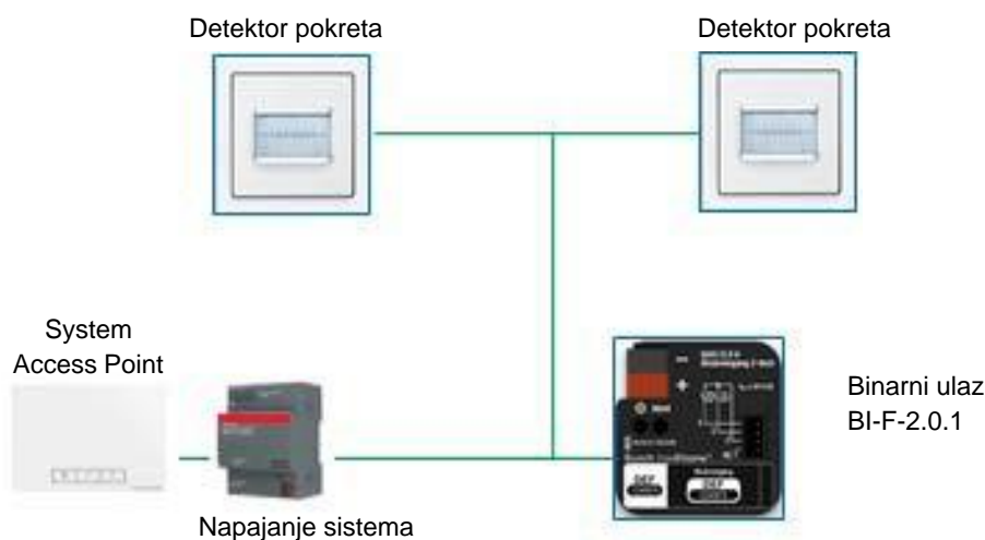
Slika. 1: Pregled sistema
